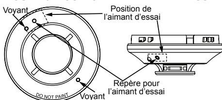
FIGURE 3. POSITION DE L'AIMANT D'ESSAI
