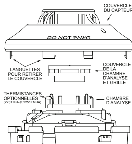
FIGURE 4. ASSEMBLAGE DU CAPTEUR
